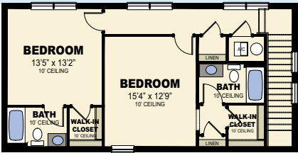
OPTIONAL UPPER ENSUITES
